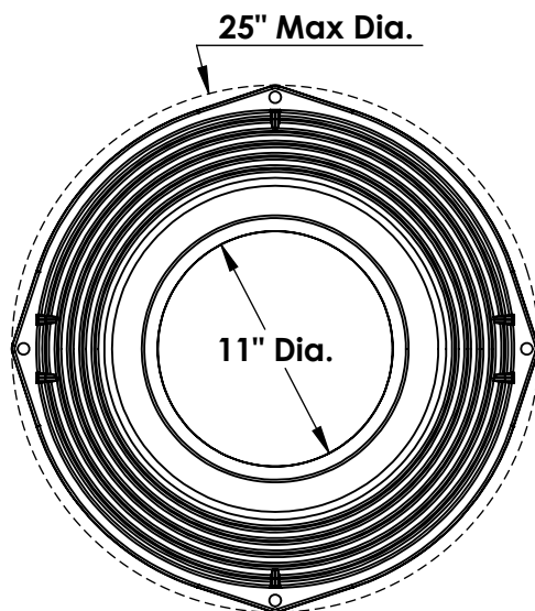
View A-A
